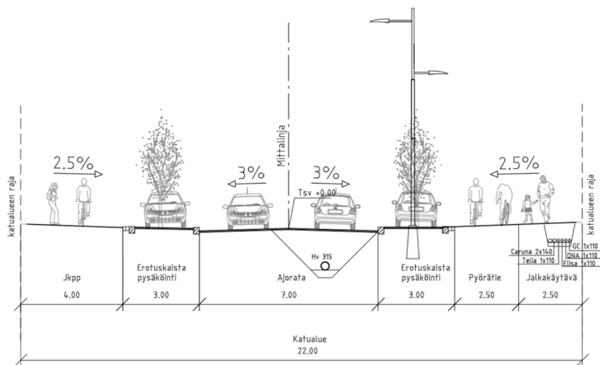
Kokoajakadun tyypipoikkileikkaus (Puistometsäntie), Kuva: WSP Finland Oy
